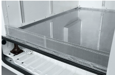
㉕ エアダム(サイドドア用) サイドドア下部からの冷気の流出を抑えます。
