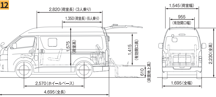
リフト付バン 標準フロア・2WD (3BF-TRH200K-VTASTL)
