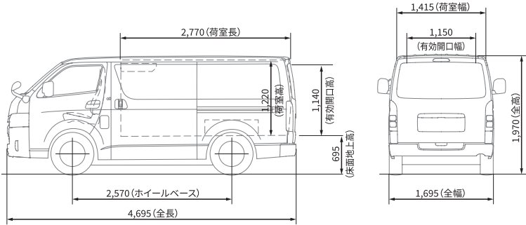
寸法図 (単位:mm)
