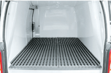
21 スノコ(樹脂製) 耐食性に優れたスノコです。
